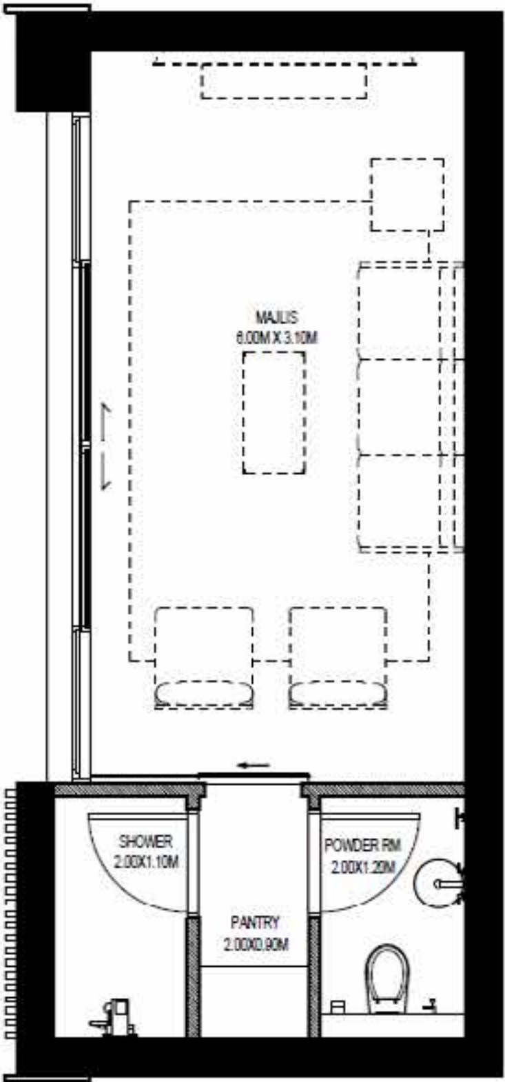
MAJLIS LAYOUT
